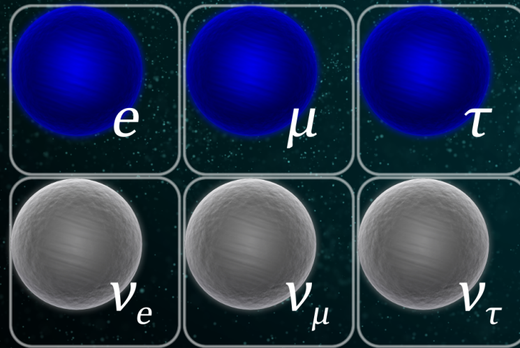
Leptons
